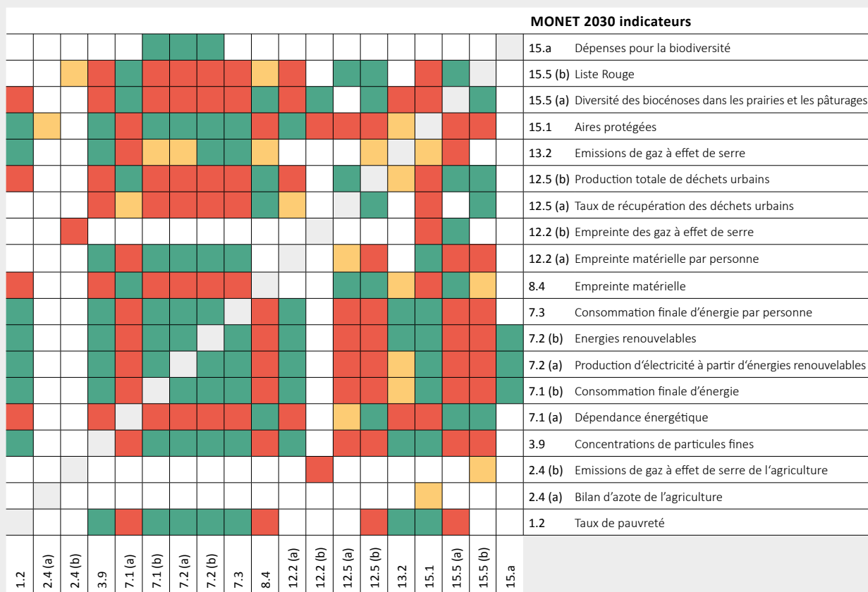
Graphique 6: Corrélations (synergies et conflits d'objectifs) entre les sous-objectifs prioritaires des ODD pour la Suisse, calculées via une analyse de corrélation de rang de Spearman.
